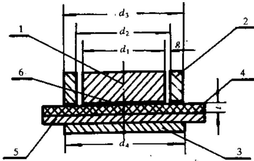
图 B.3.3 试件与电极配置
