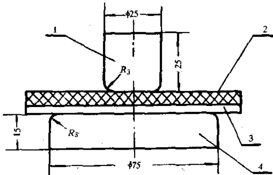
图 A.3.2 试件与电极配置
